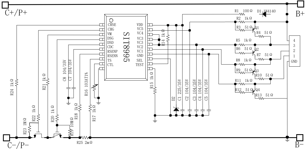
图 9 SIT8995 典型应用图（4 串同口应用）
