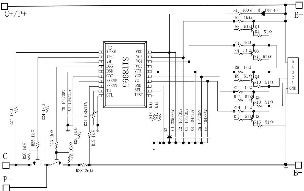
图 10 SIT8995 典型应用图（5 串分口）
