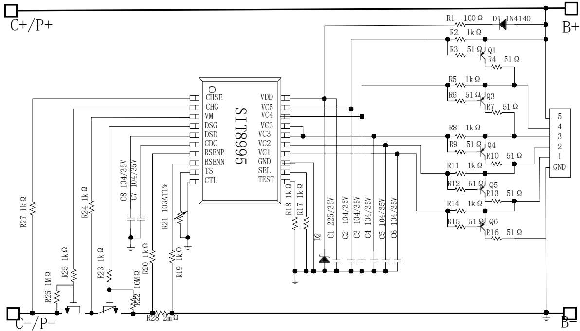
图 8 SIT8995 典型应用图 (5 串同口)
