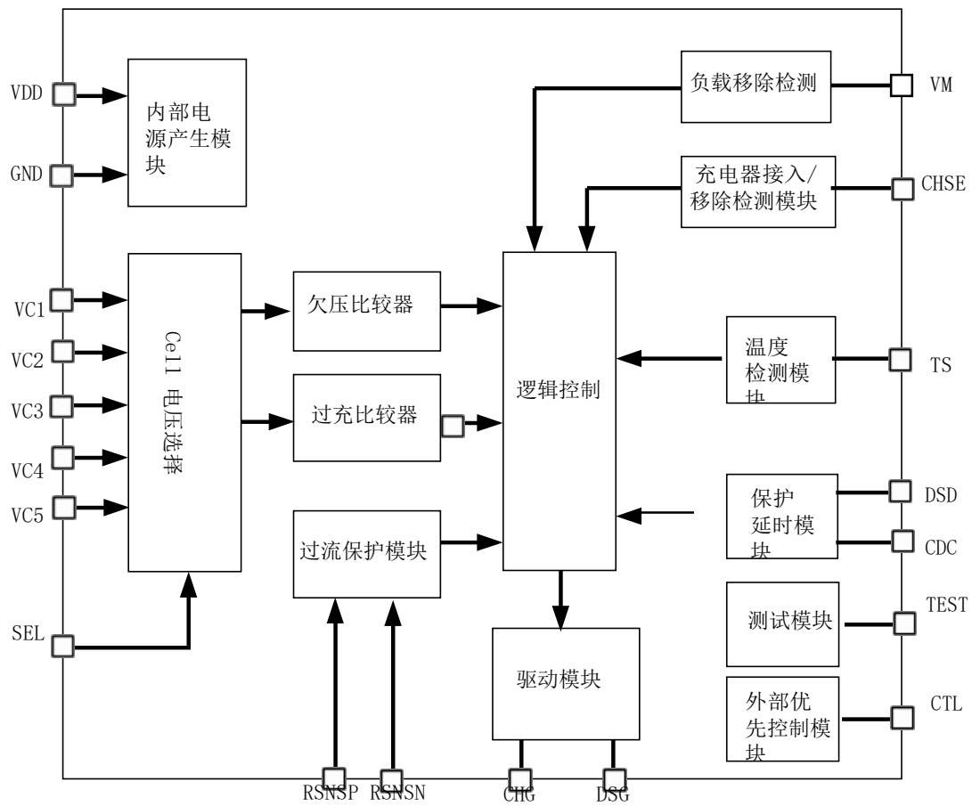
图 1 SIT8995 系统框图
