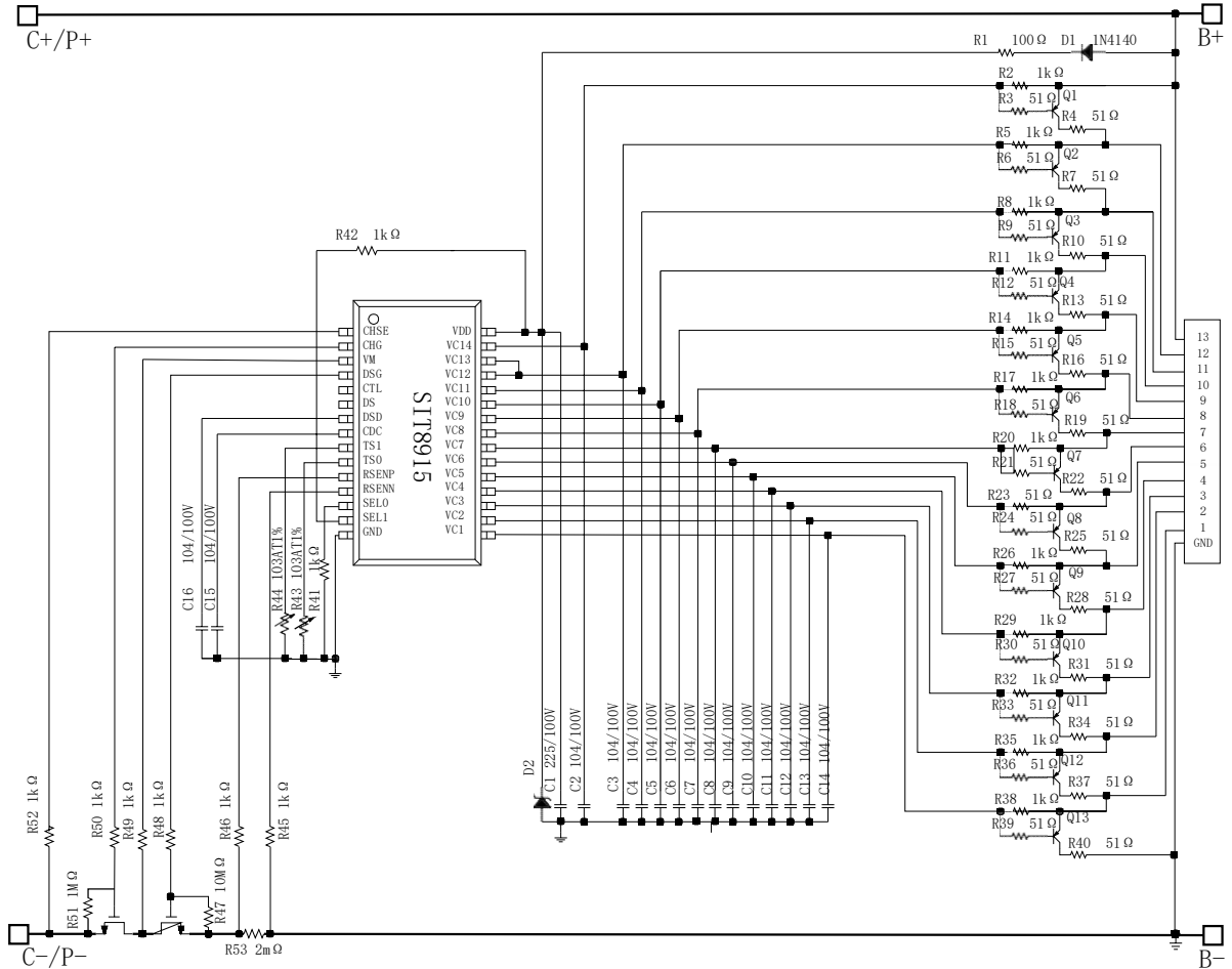
图 9 SIT8915 典型应用图（13 串同口应用）
