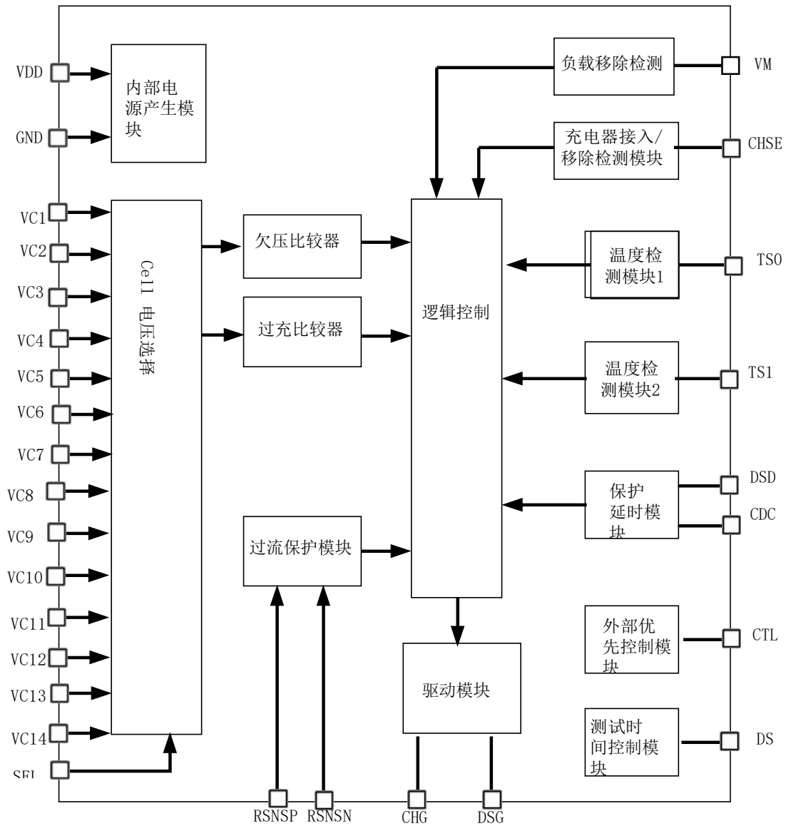
图 1 SIT8915 系统框图
