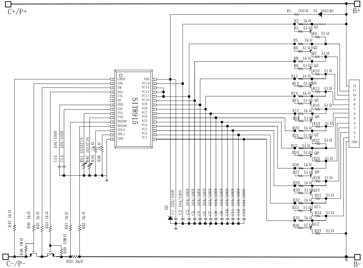
图 10 SIT8915 典型应用图（12 串同口应用）
