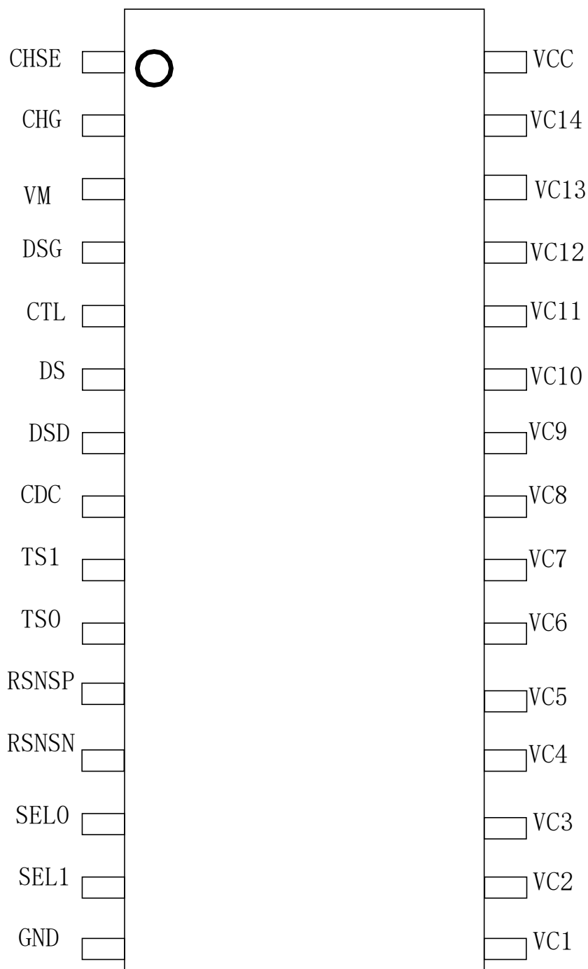
图 2 SIT8915 管脚图
