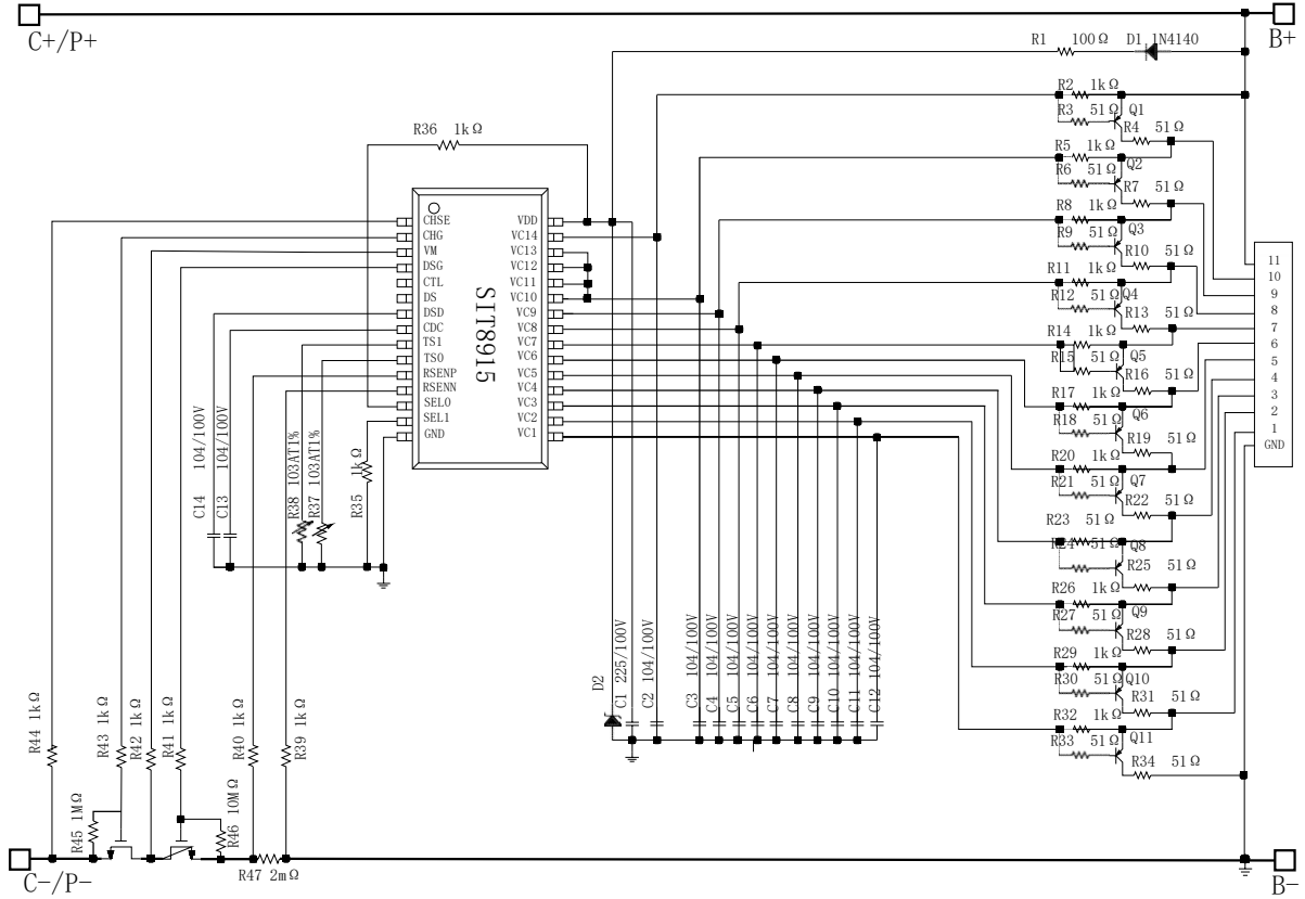
图 11 SIT8915 典型应用图（11 串同口应用）
