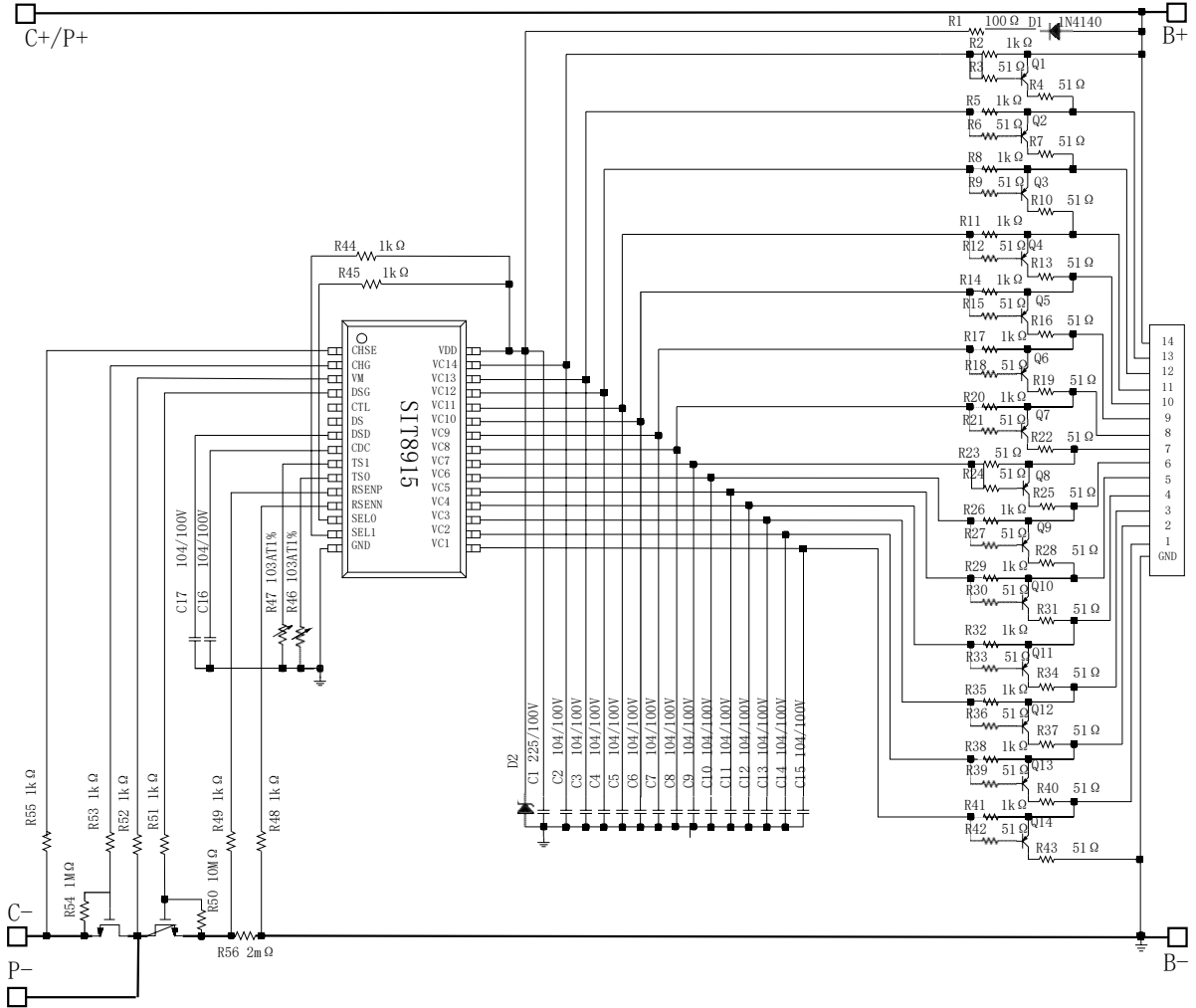
图 12 SIT8915 典型应用图（14 串半分口）
