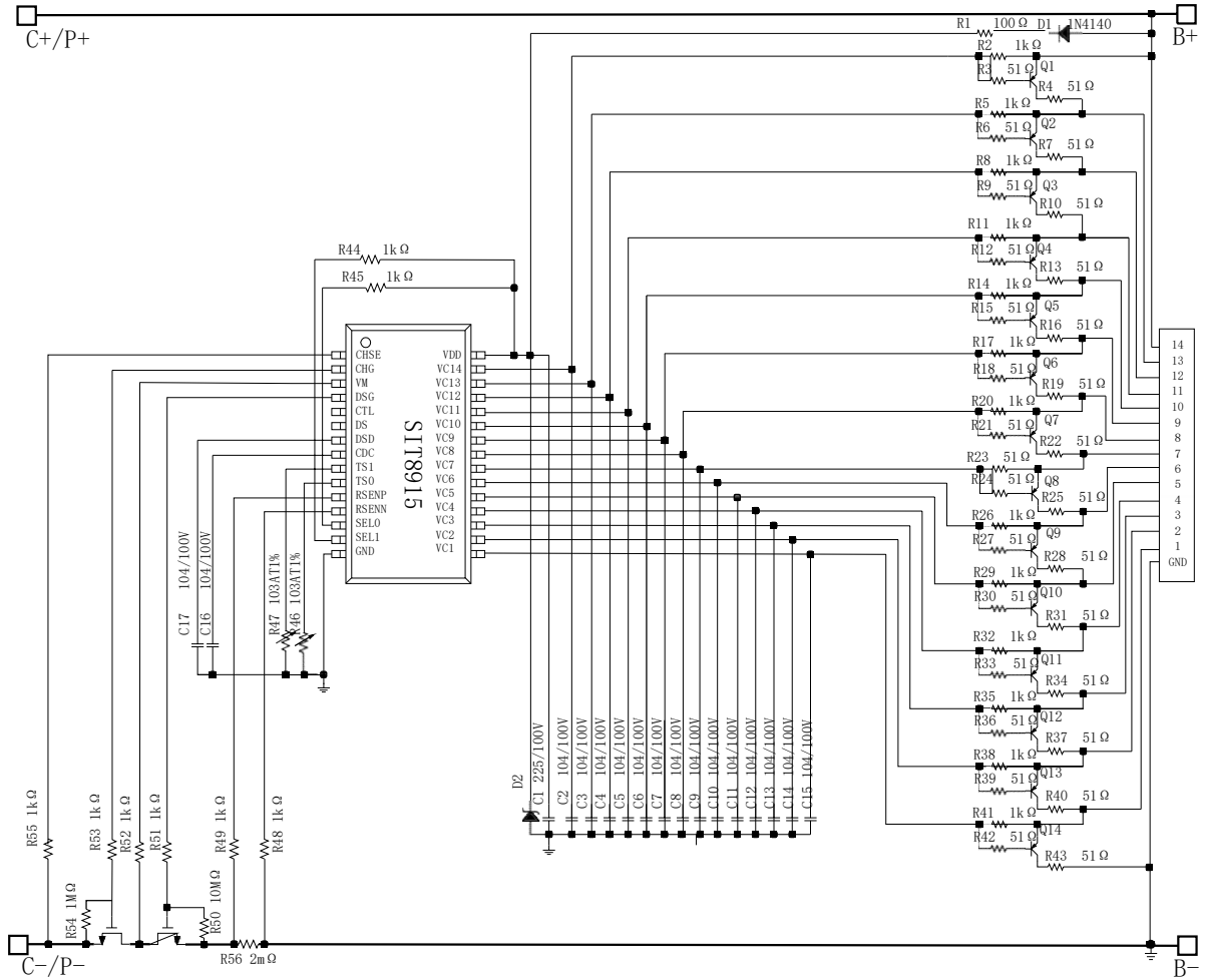
图 8 SIT8915 典型应用图 (14 串同口)
