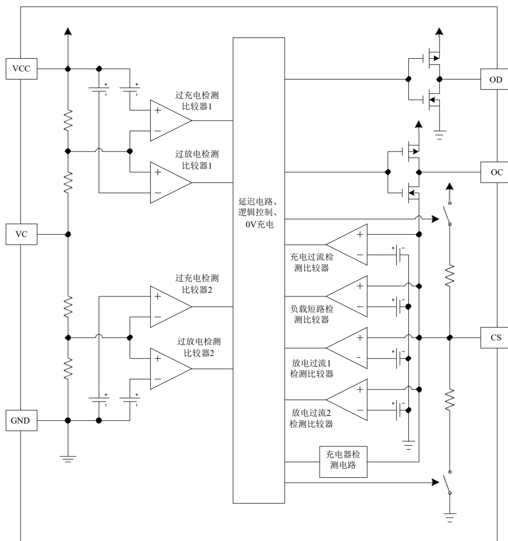
图 2. 功能框图
